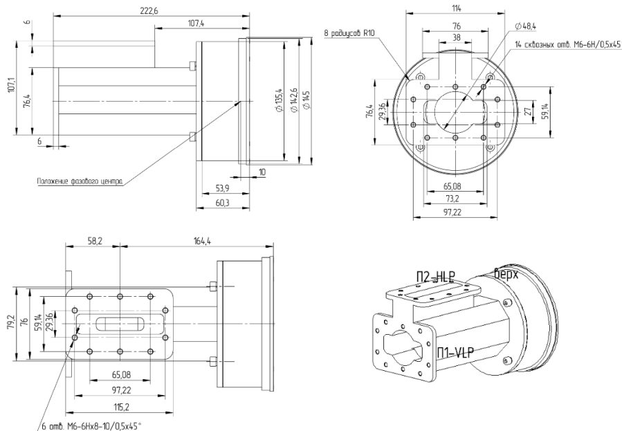
Рисунок 1 – Габариты изделия.
